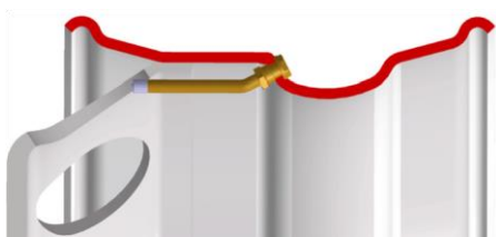
DCW-G1 – старое поколение Колесо с внутренним вентиляем
